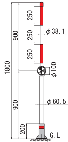
アンカーボルト C-1060
