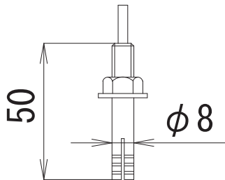
アンカーボルト C-850
