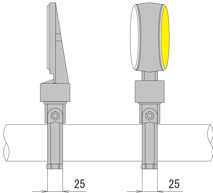
NP-100S (片面)
