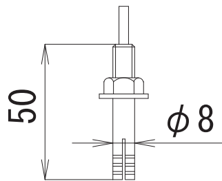
アンカーボルト C-850
